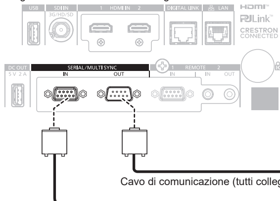
Collegamento dei terminali del proiettore da sincronizzare
