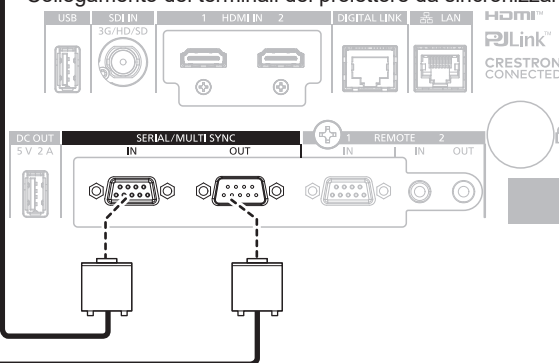
Collegamento dei terminali del proiettore da sincronizzare
